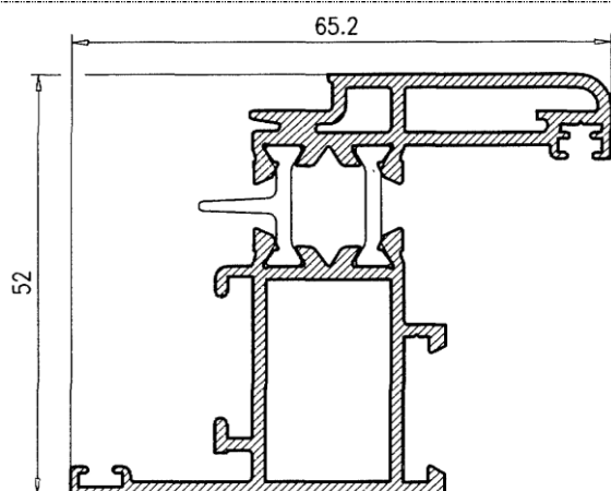
Hoja Enrasada Ventana 25380
