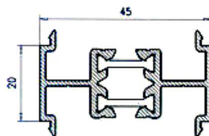
Unión Marcos 25003
