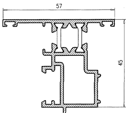
Marco Ventana 25280
