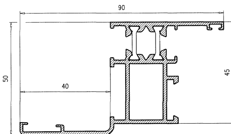
Marco solape con resalte 25281
