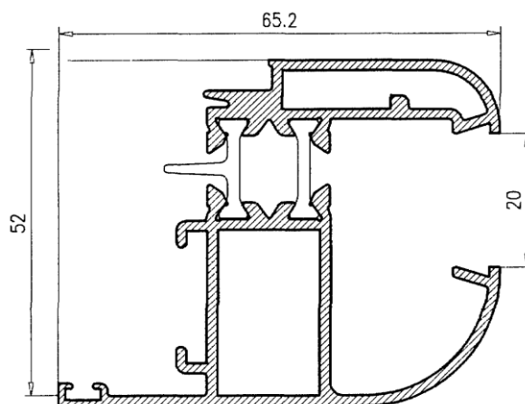
Hoja Ventana s/junq 25382
