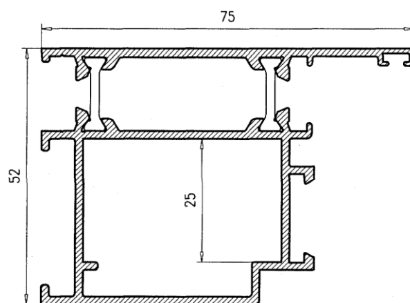
Marco Puerta Enrasado 26281
