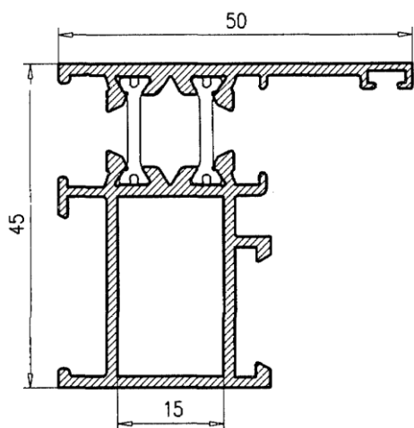
Marco Ventana 25280
