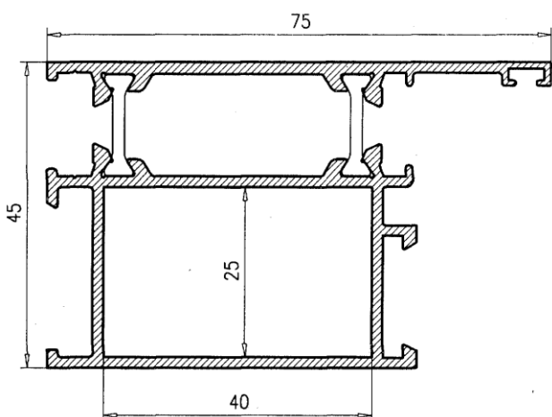
Marco Puerta 26280
