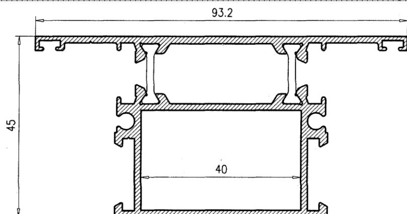
Pilastra Puerta 26580
