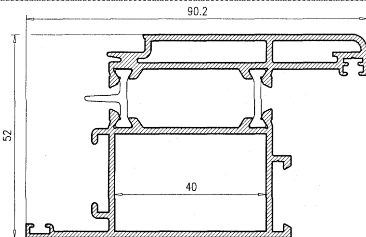
Hoja Puerta Enrasada 26380
