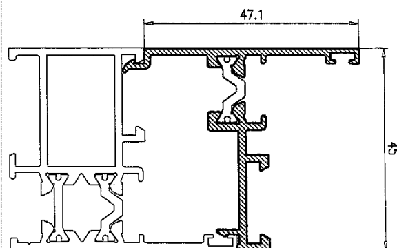
Inversor de marco 25384
