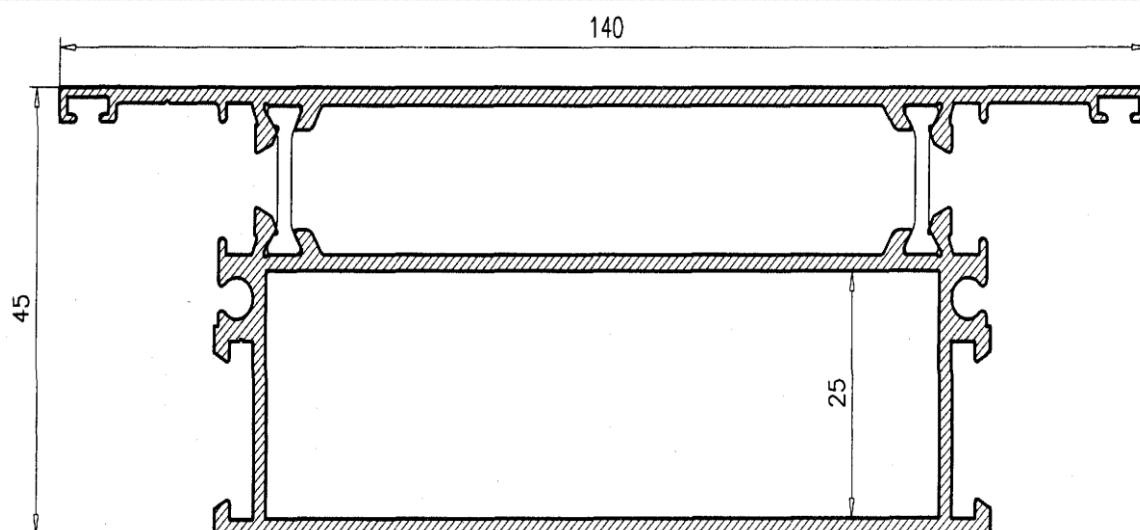
Pilastra Zócalo 26476
