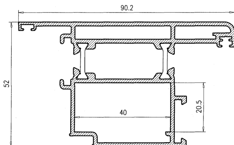
Hoja Apertura Exterior 26581
