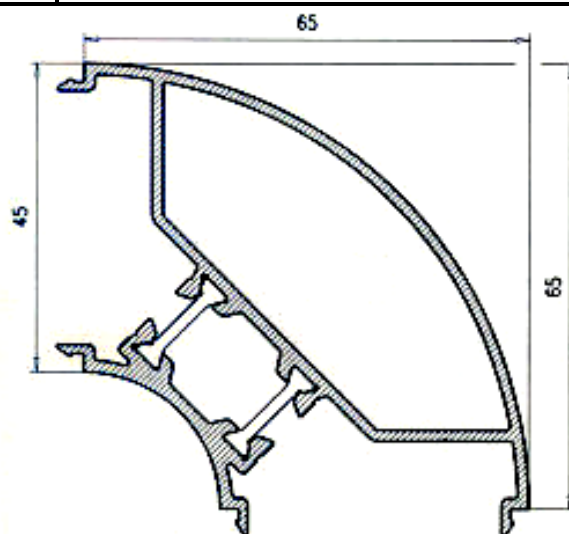
Esquinero 45 25092
