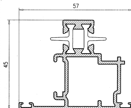
Perfil Pivotante 25284
