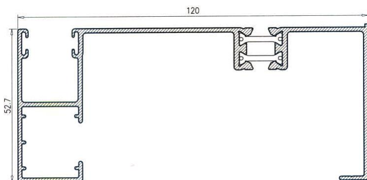
Guía con solape 25120
