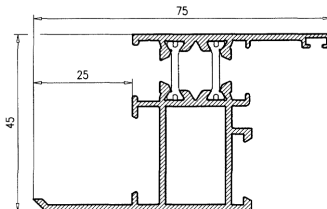
Marco Ventana c/premarco 25282
