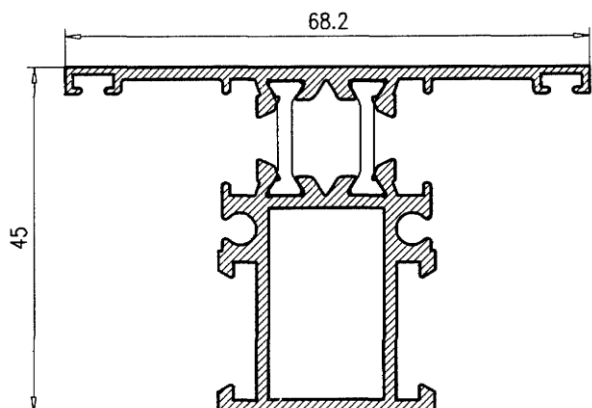
Pilastra Ventana 25583
