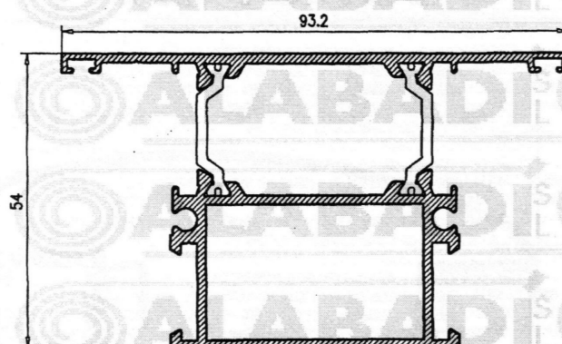
Pilastra Puerta 55580
