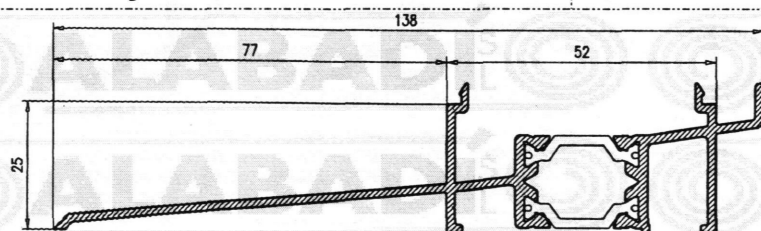
Vierteaguas 54282
