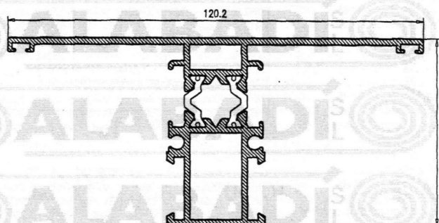
Pilastra Ventana 54584
